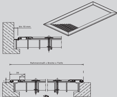
Lichtschachtdeckung ▲
